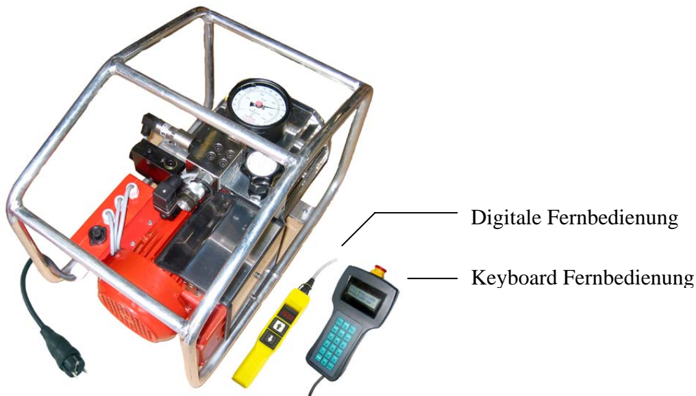
Elektro-Aggregat, Typ EA 18
